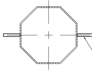
A - A KESİTİ SECTION A-A
