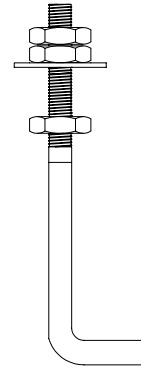
ANKRAJ CIVATASI ANCHOR BOLT
